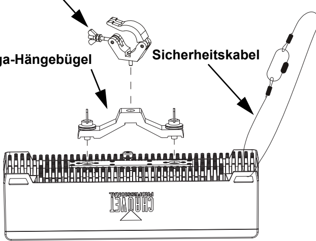
Montage über Kopf
